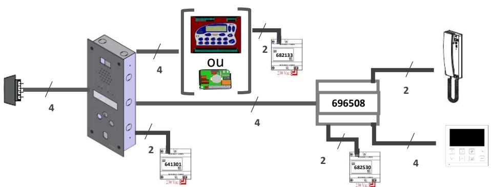
Décodeur d'étage Ref.696508
